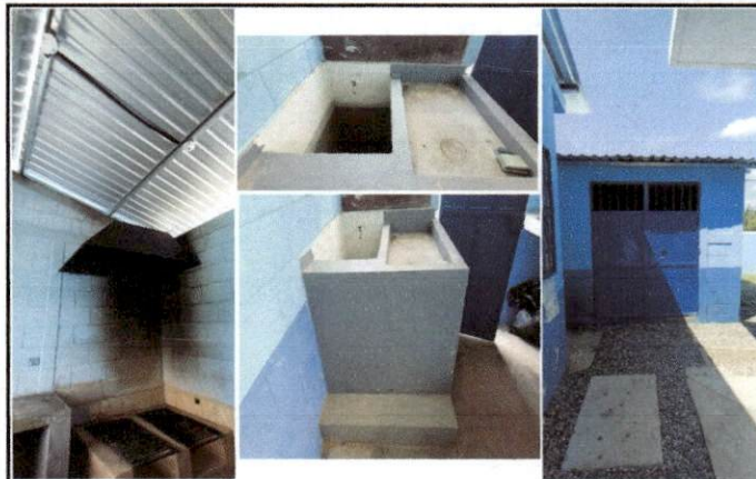
Foto 2: Polletón de 2 parrillas con su extractor de humo instalado. Reparación de pila. Drenaje de la pila al exterior instalado.
